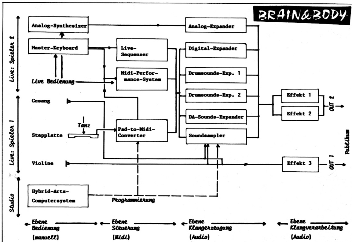
Skizze 1: Schaltbild des Brain & Body Projekts
