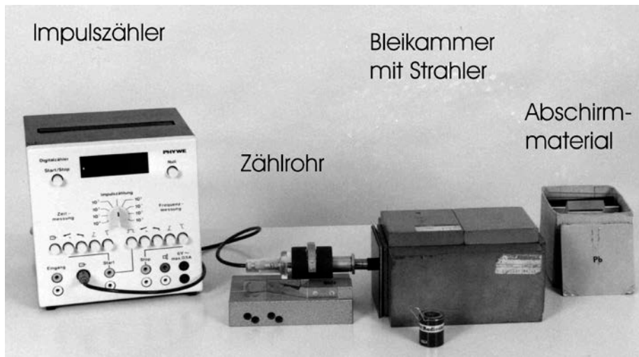
Messung der Reichweite radioaktiver Strahlung
