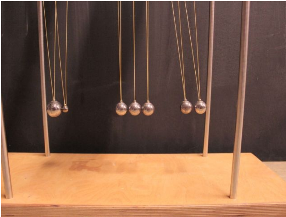
Abb. 2: Zwei von 5 Kugeln sind ausgelenkt.
