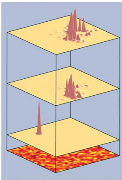
Abb. 2: Numerisch berechnete Aufenthaltswahrscheinlichkeiten von drei lokalisierten Exzitonenzuständen (im unten dargestellten Unordnungspotential) mit leicht unterschiedlichen Emissionswellenlängen.
