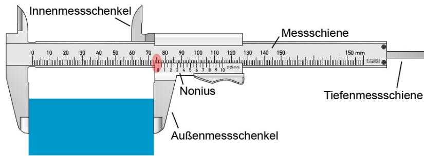
Abb. 2: Messschieber 2 zur Messung von Außenmaßen (Beispiel: blauer Quader), Innenmaßen und Tiefenmaßen. Auf der Messschiene werden die ganzen Millimeter abgelesen (nächster Skalenswert links neben der „0“ des Nonius , hier 75 mm). Auf dem Nonius erfolgt die Ableseung des Nachkommawertes (Abb. 3).
