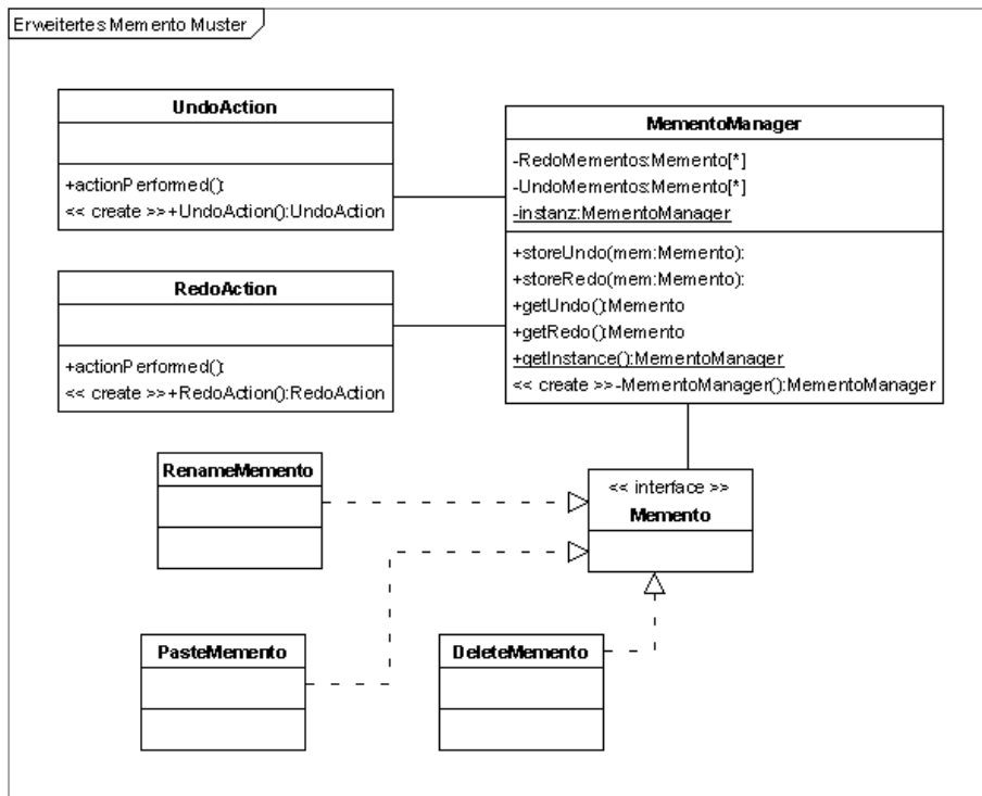
Abb. 4.: Abstraktes, angepasstes Memento – und Singleton – Muster
